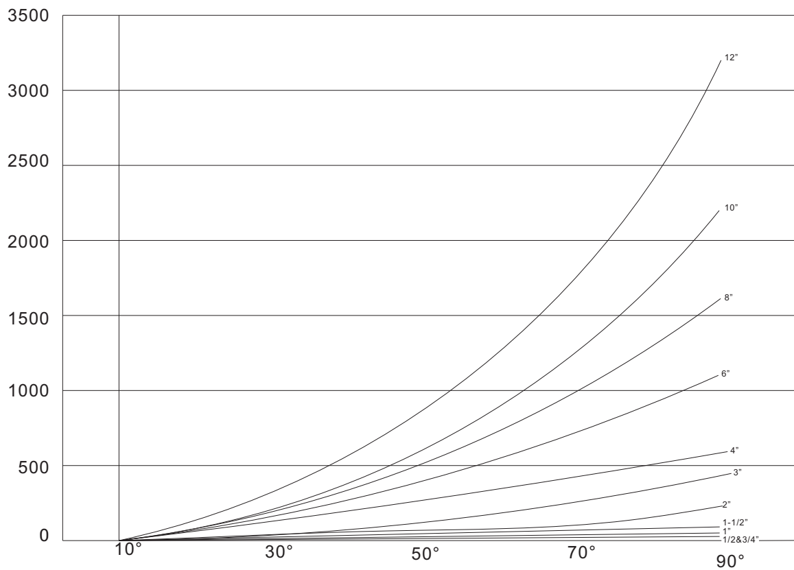
阀门开闭、调节扭矩 Torque Data Unit:N•M 表4 Table4
