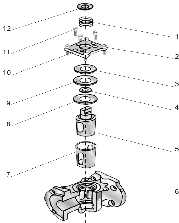
阀本体结构 Configuration of Body
